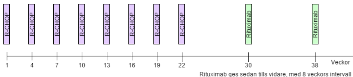
Figur 3. Behandlingsöversikt R-CHOP-21 \times 8 + Rituximab-underhåll
